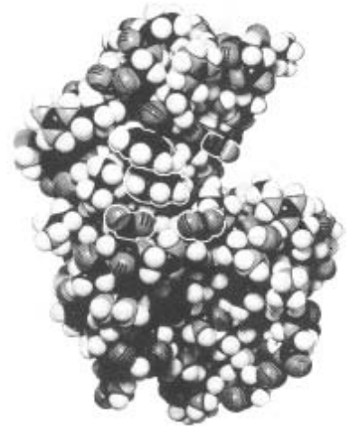
Kugelmodell eines Enzyms (jede Kugel repräsentiert ein Atom)
